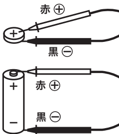
直流電圧測定
